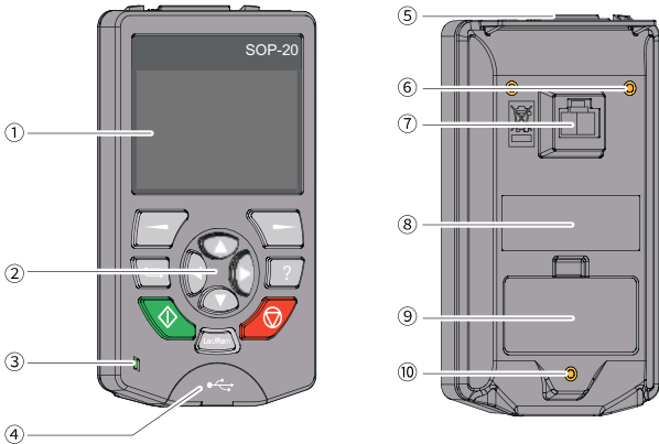
图3-12 SOP-20-CP各部分组成示意图
