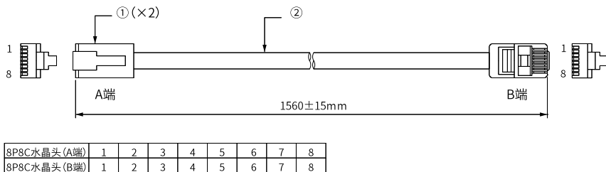
图3-13 外引操作键盘连接线缆示意图
