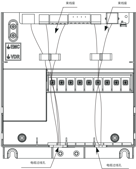
图2-12 控制线线缆走线示意图
