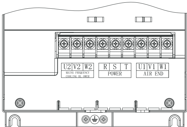
图2-4 CP200-4T11-H~CP200-4T15-H主回路端子分布示意图
