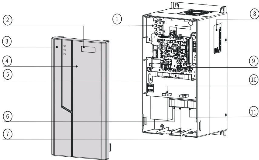
图1-3 部件示意图
