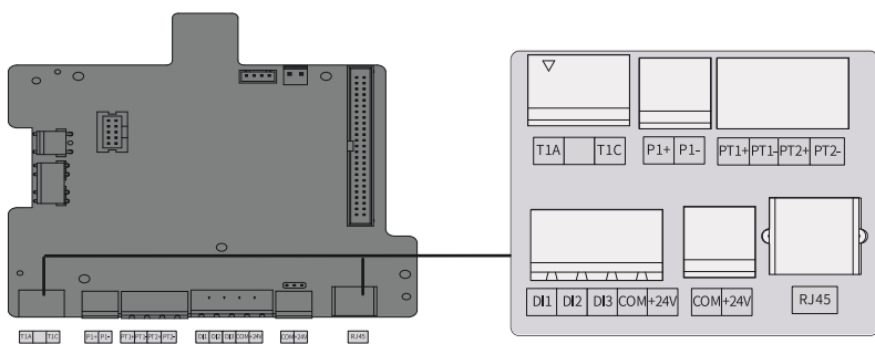
图2-6 控制端子分布示意图
