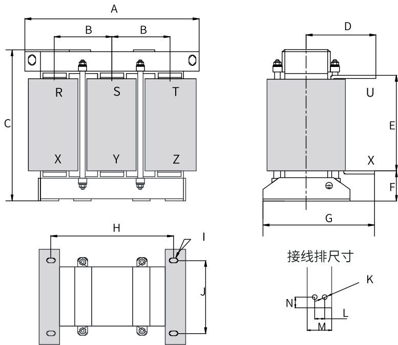
图1-12 800A-1000A输入电抗器尺寸图
