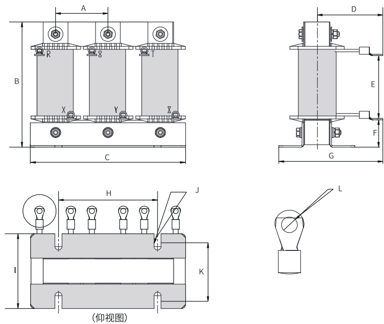
图1-8 50A(0.28mH) / 60A输入电抗器尺寸图
