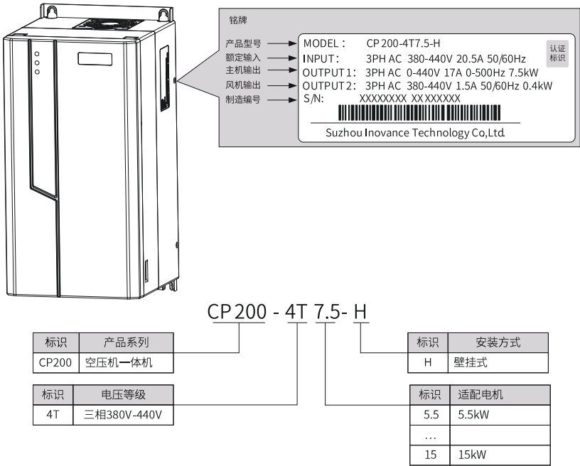
图1-1 产品铭牌与型号说明
