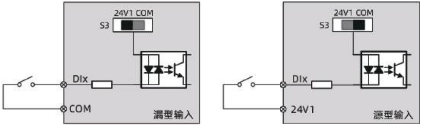
图2-9 数字输入端子源型漏型接线示意图
