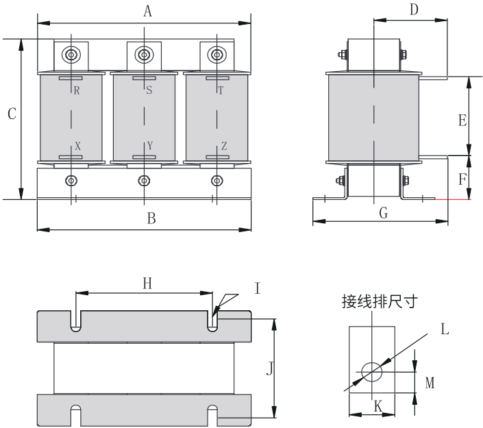
图1-9 80A / 120A输入电抗器尺寸图
