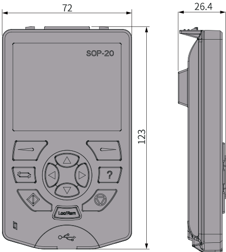
图3-11 SOP-20-CP尺寸图（单位：mm）
