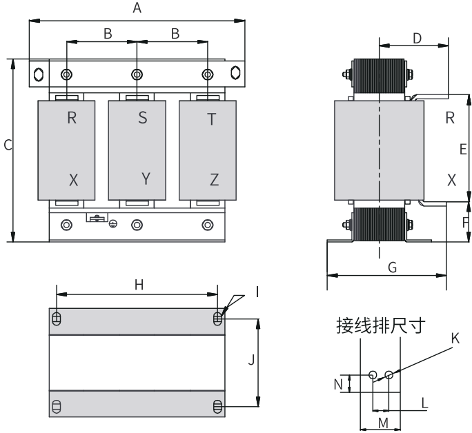
图1-11 490A / 660A输入电抗器尺寸图
