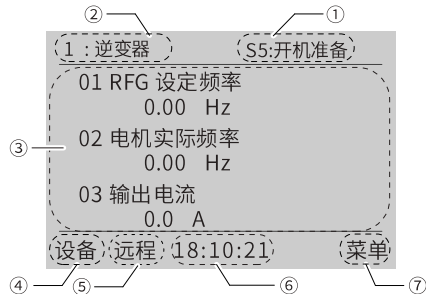
图3-14 SOP-20-CP界面显示举例
