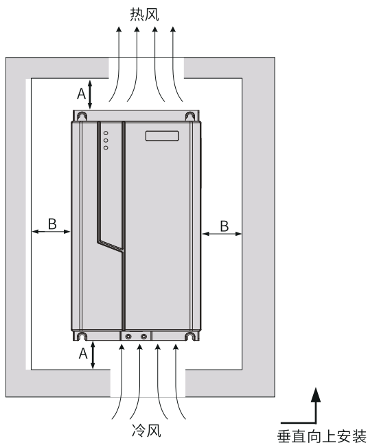
图2-2 安装空间要求
