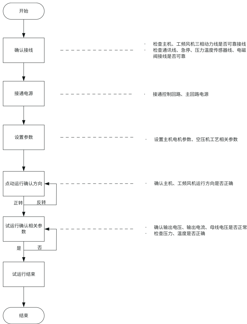
图3-2 调试流程图
