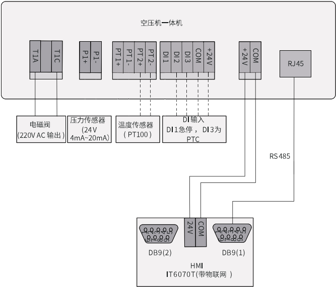
图2-7 控制端子接线示意图
