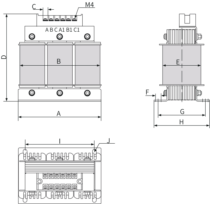
图1-6 10A~15A输入电抗器尺寸图
