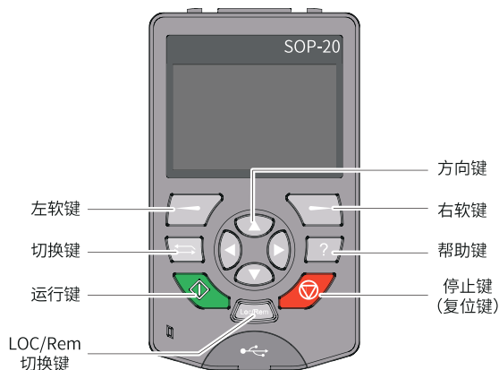
图3-15 各按键位置示意图
