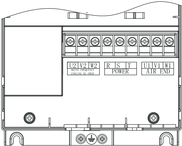
图2-3 CP200-4T5.5-H~CP200-4T7.5-H主回路端子分布示意图
