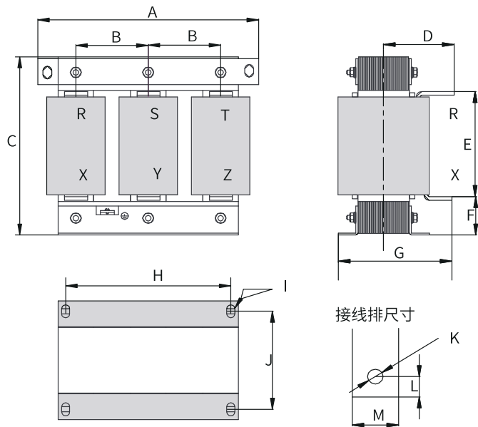
图1-10 150A-330A输入电抗器尺寸图
