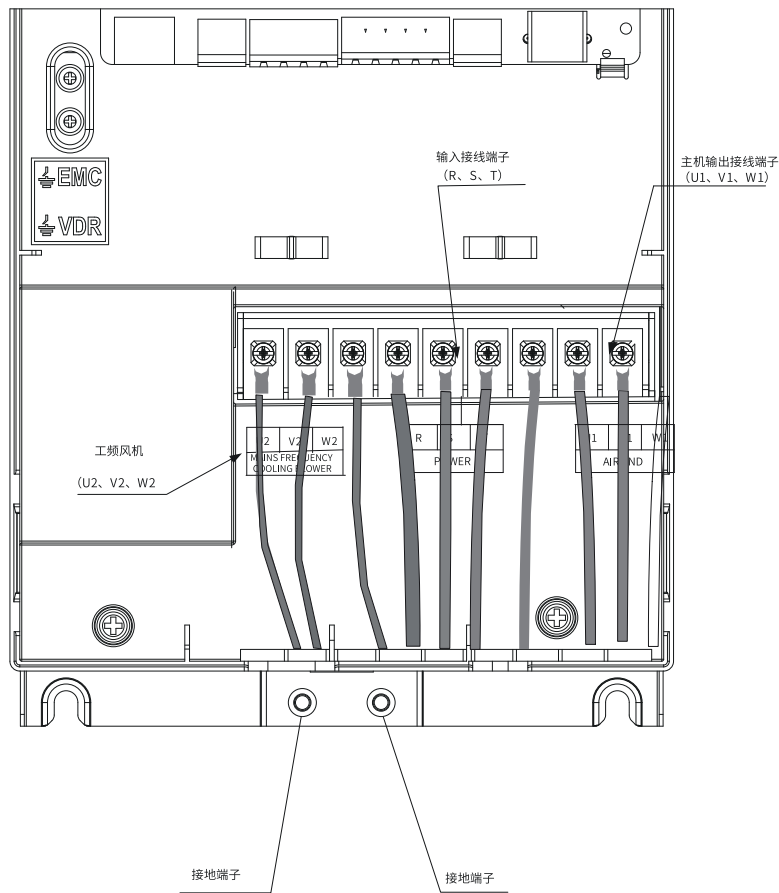
图2-11 主功率线接线示意图
