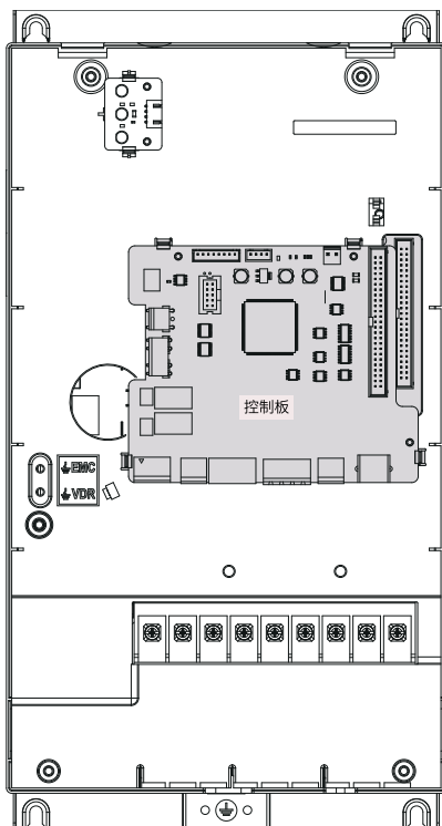
图2-5 控制板位置示意图
