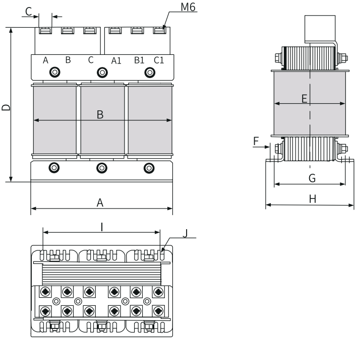
图1-7 40A / 50A(1.2mH)输入电抗器尺寸图
