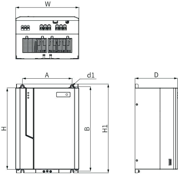
图1-2 壁挂式机型安装尺寸示意图
