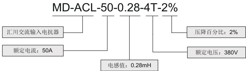
图1-5 输入电抗器型号
