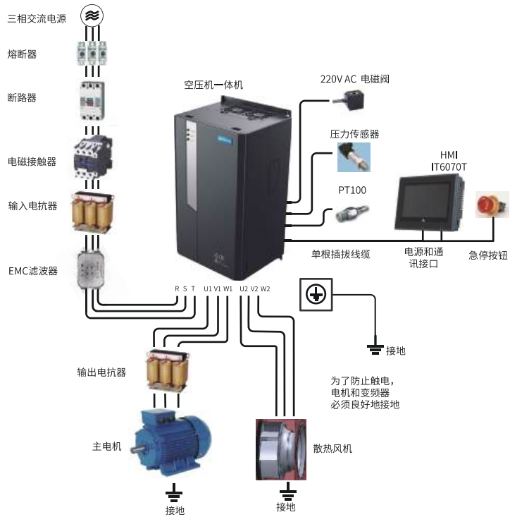
图1-4 系统构成示意图
